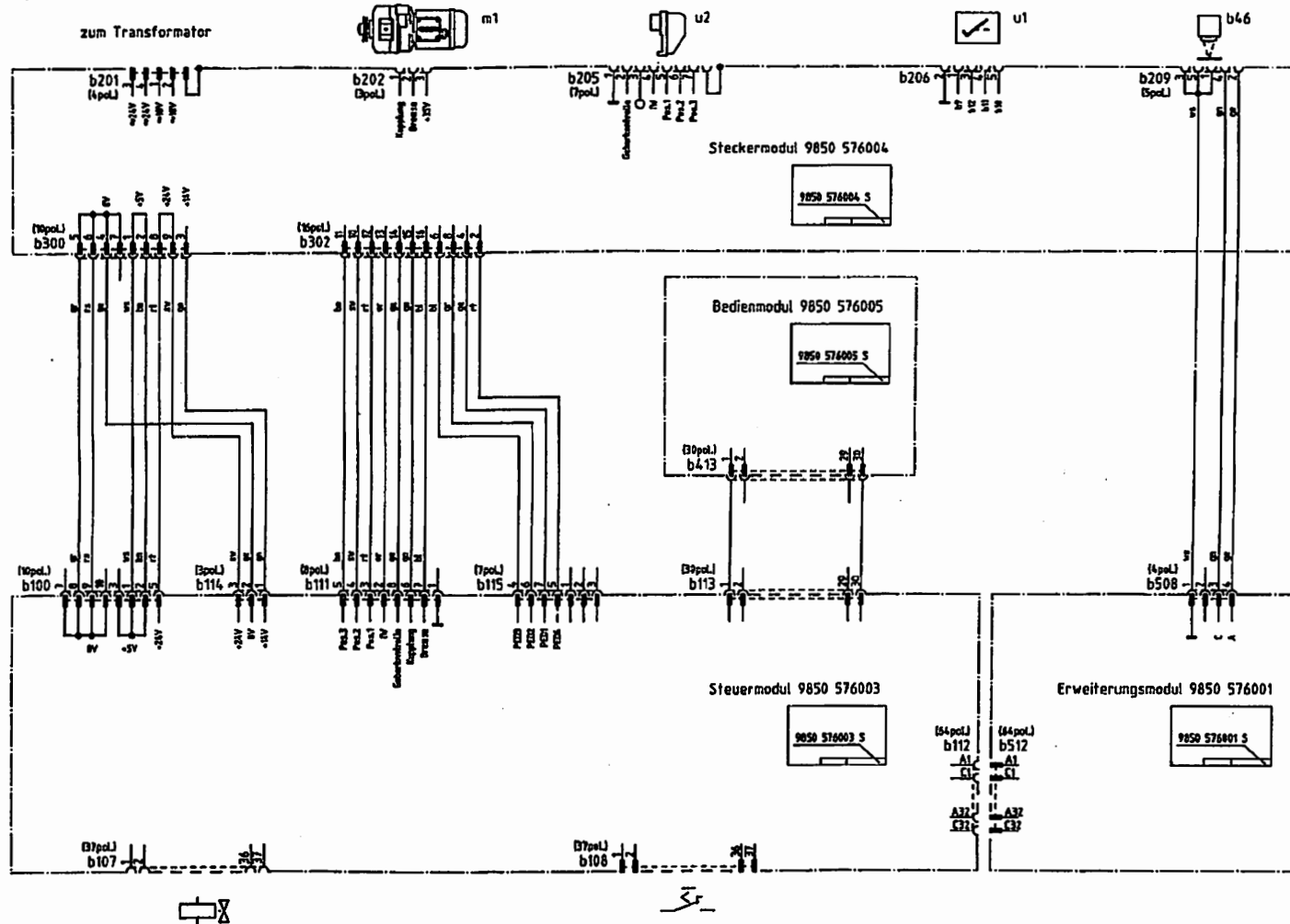
Bauschaltplan 9890 576001 B
