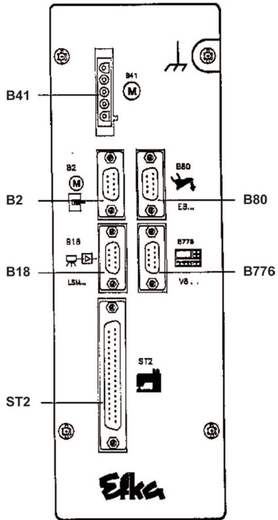
Anschlussbuchsen-ST220A
