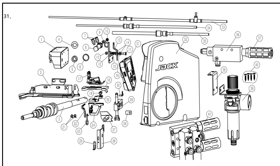
三十一、C5倒回缝专用部件/ Specific Parts
