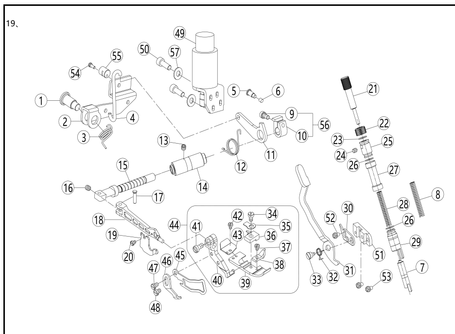
十九、抬压脚机构/Presser Foot Mechanism
