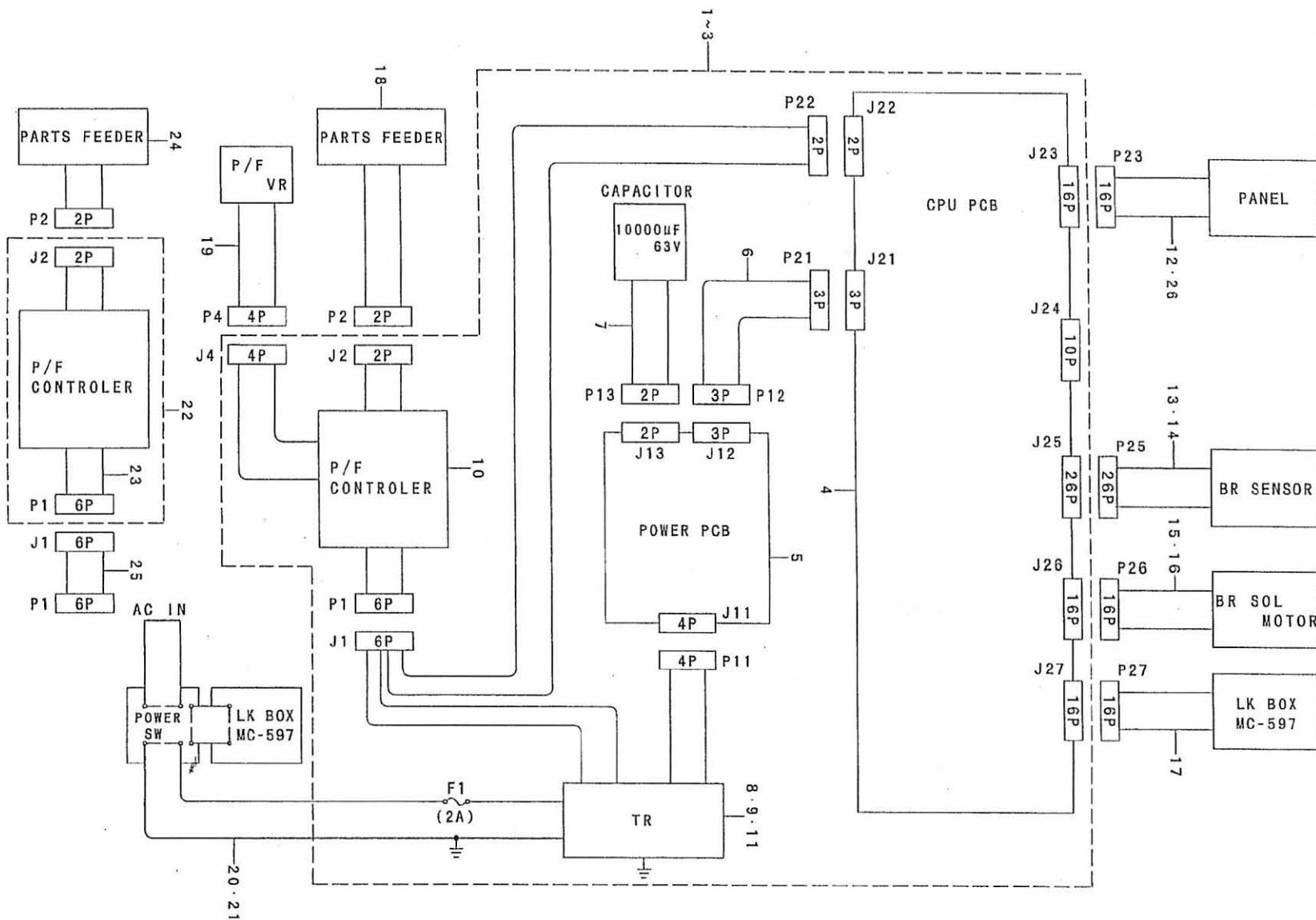
19. BR35 WIRING DIAGRAM BR35電装配線図
