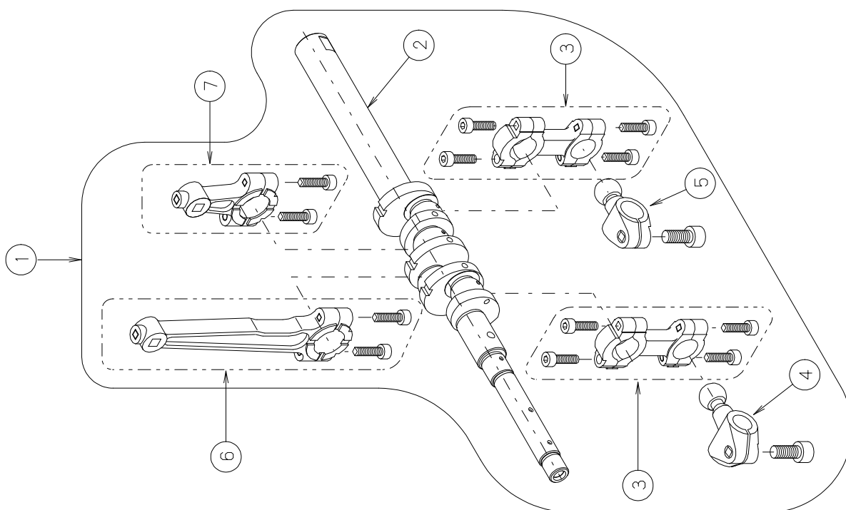
34. 主軸セット一覧表 CRANKSHAFT SET PARTS TABLE
