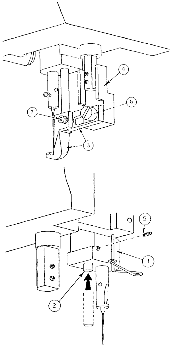
Jump Foot - fig. 19
