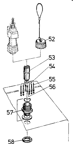
RECEPTACLE IN SWITCH-BOX (TOP VIEW) STECKDOSE IM SCHALTKASTEN (DRAUFSICHT)
