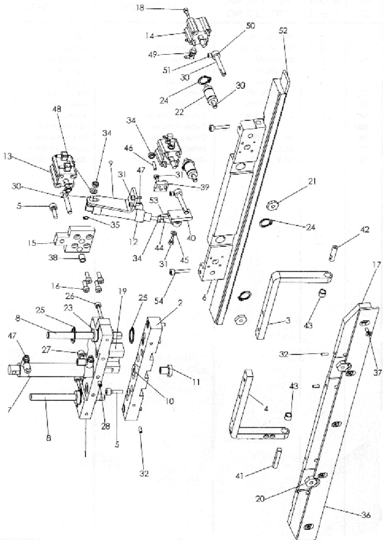
Einlegestation - lang
