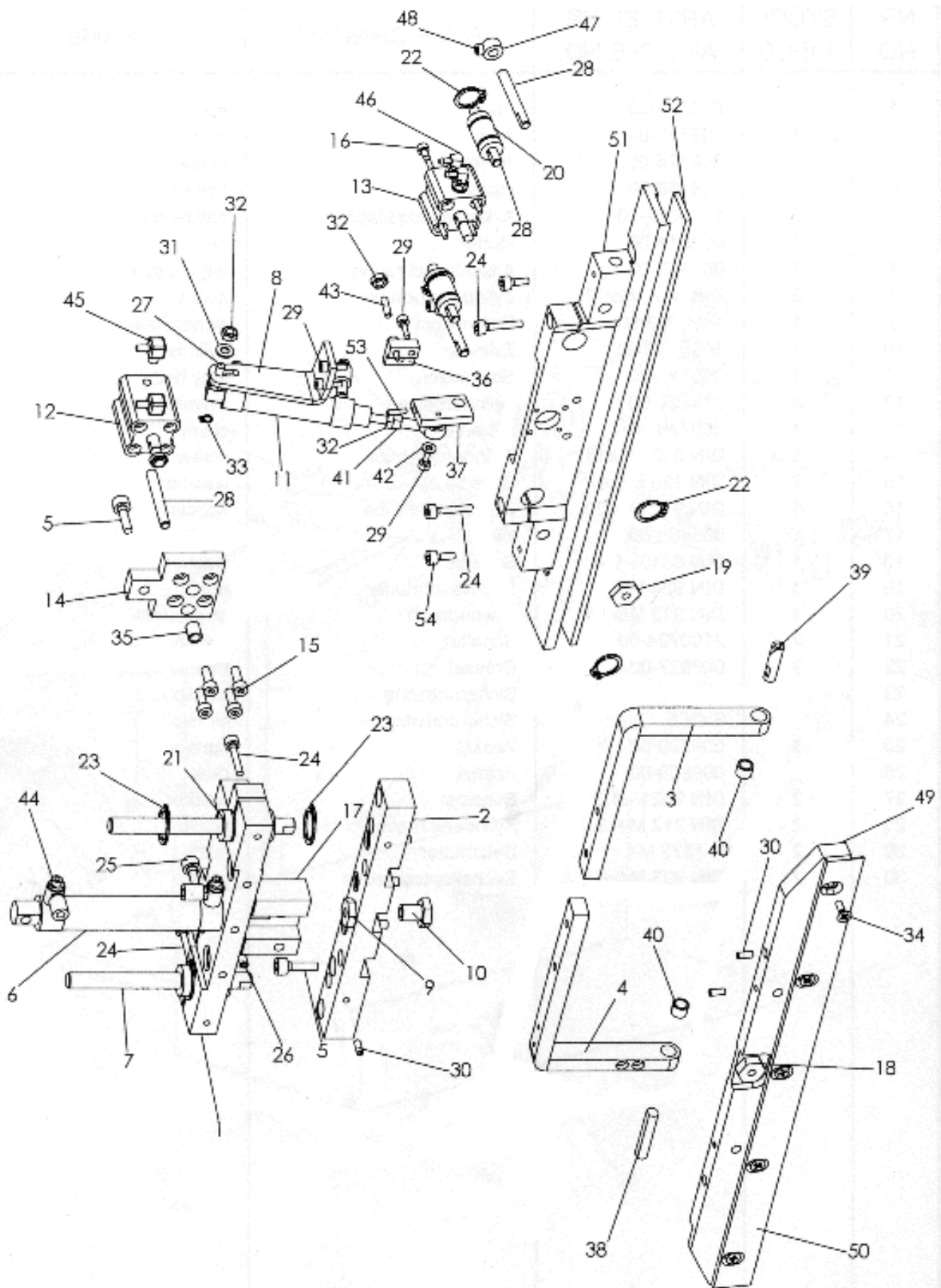
Einlegestation - kurz
