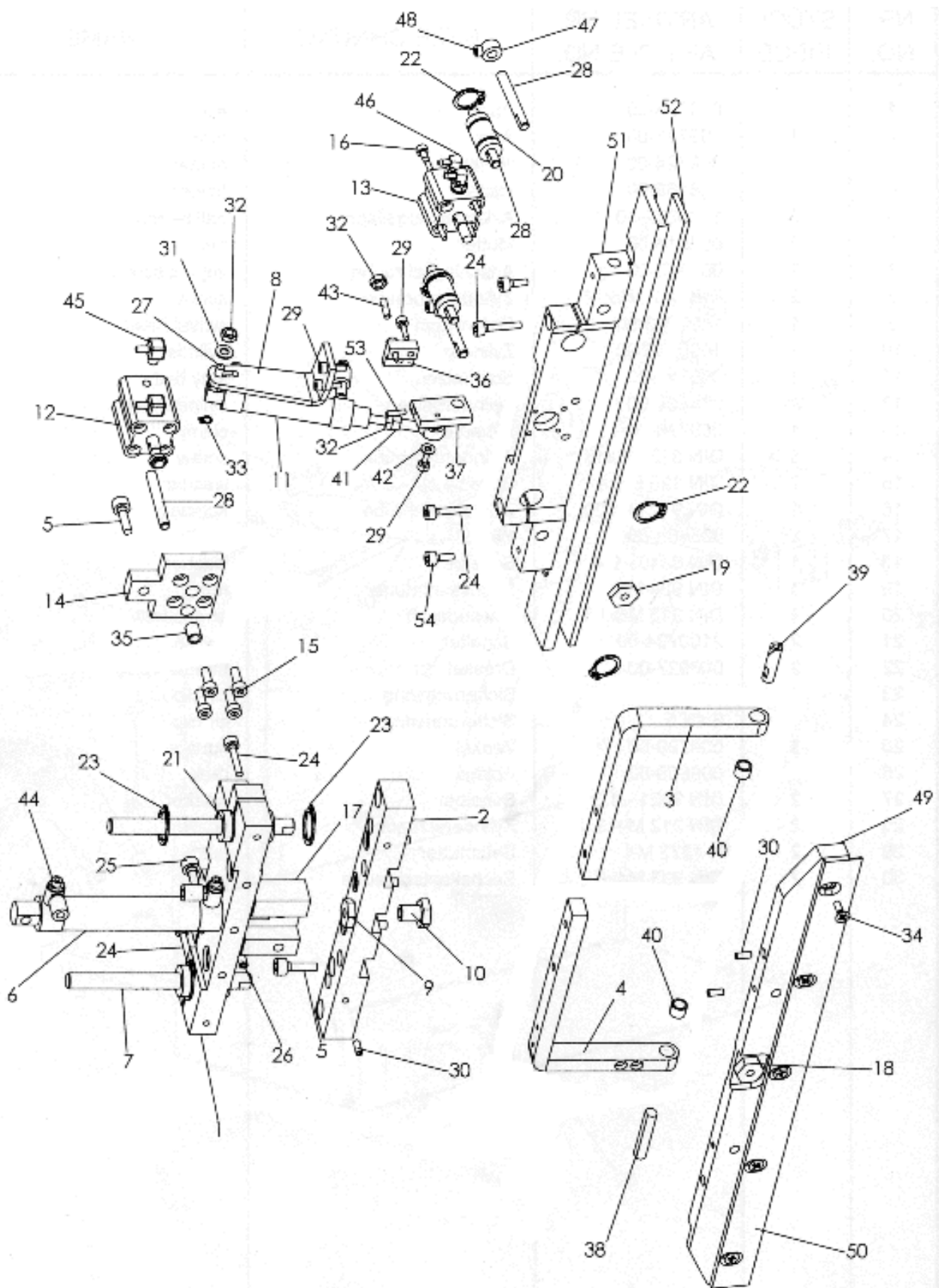
Einlegestation - kurz
