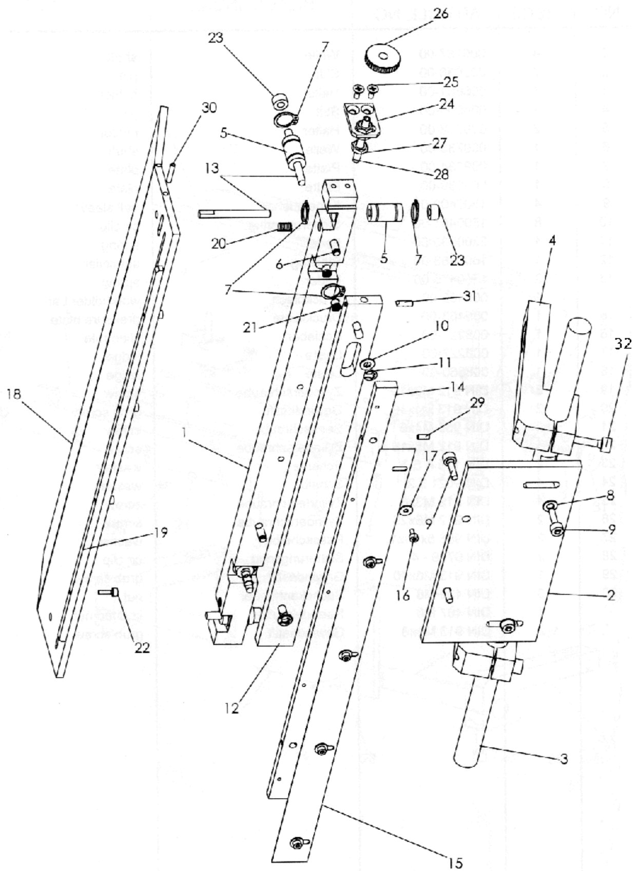
Einlegetisch - lang
