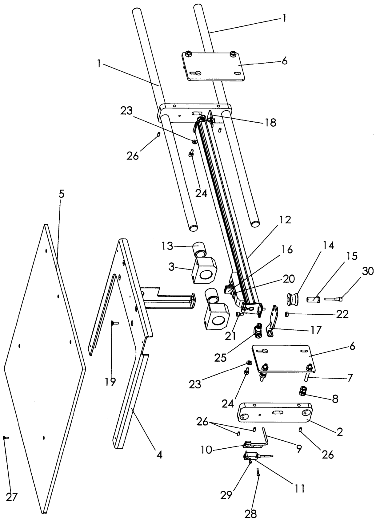
Schiebetisch
